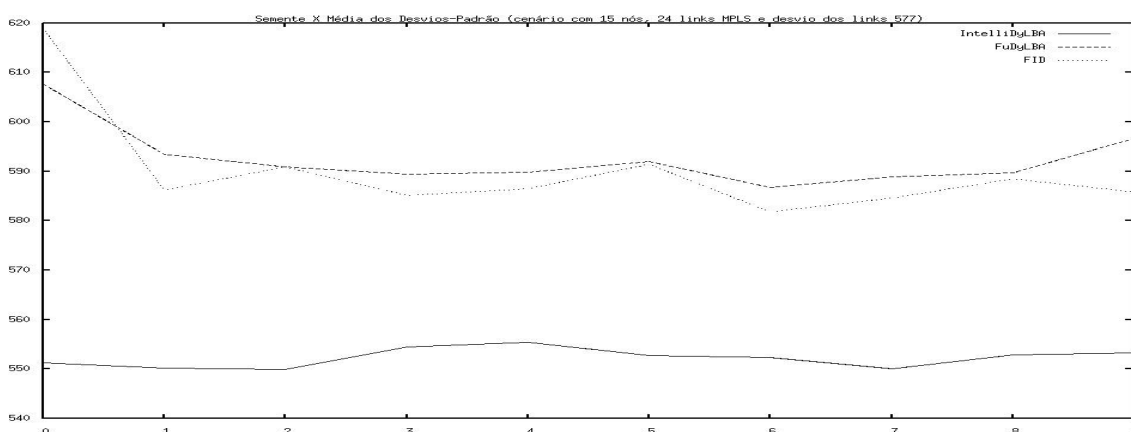
Figura 5.5. Média dos desvios padrão das bandas residuais dos enlaces ao longo dos experimentos da topologia 3.
