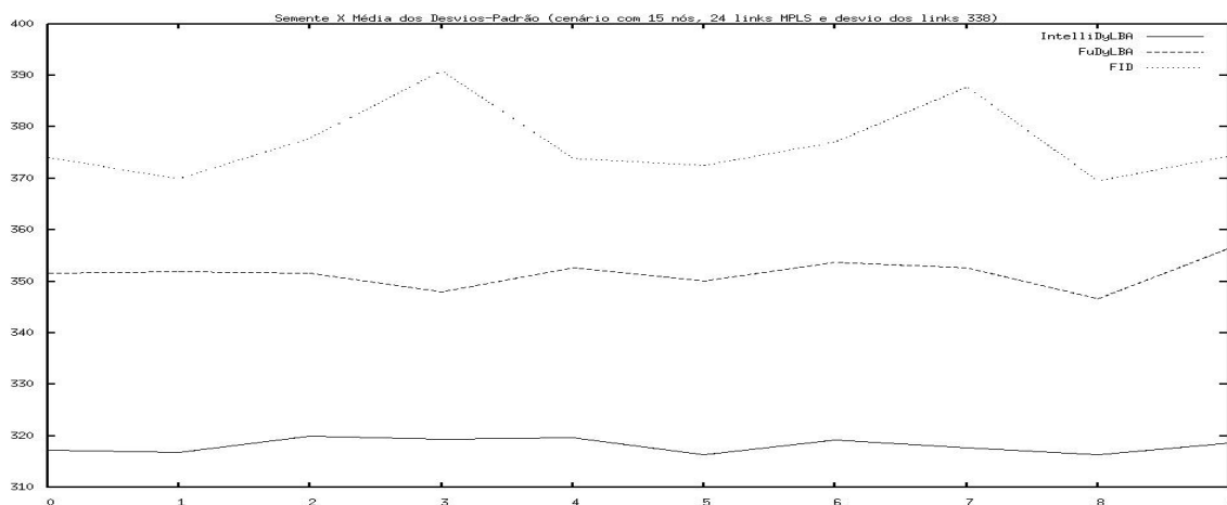
Figura 5.4. Média dos desvios padrão das bandas residuais dos enlaces ao longo dos experimentos da topologia 2.
