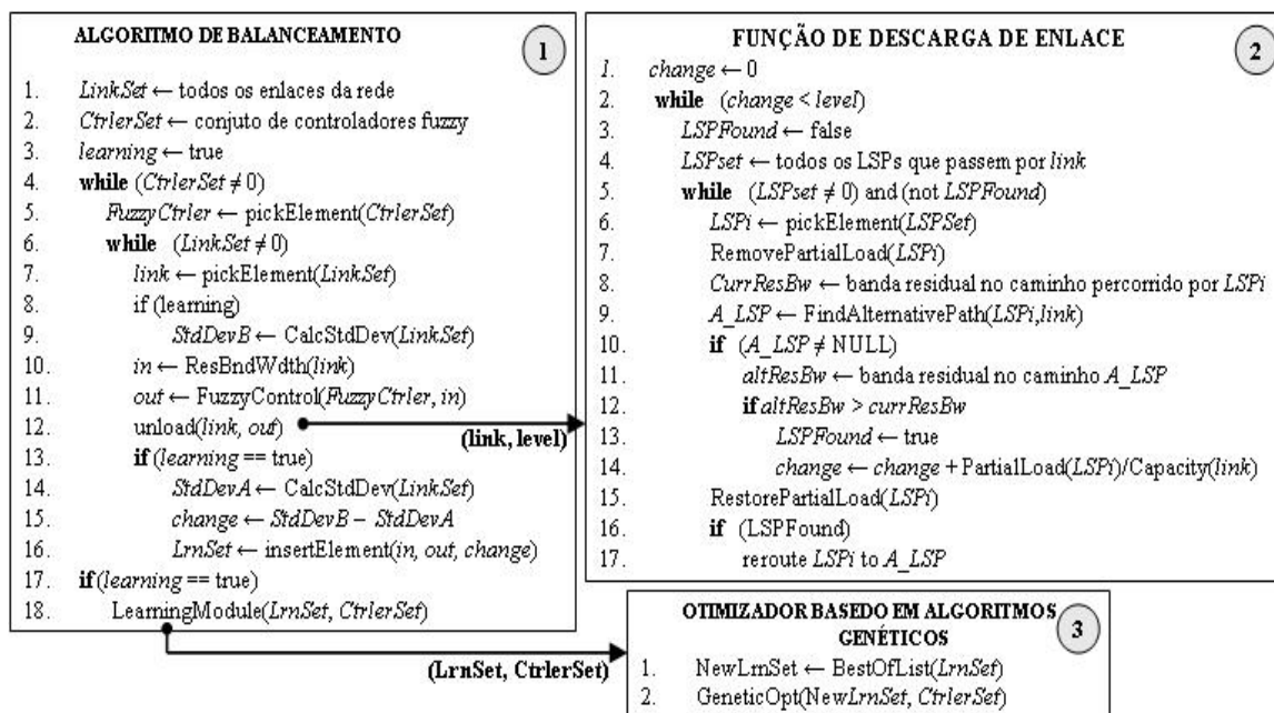
Figura 4.1. Pseudocódigo do IntelliDyLBA.
