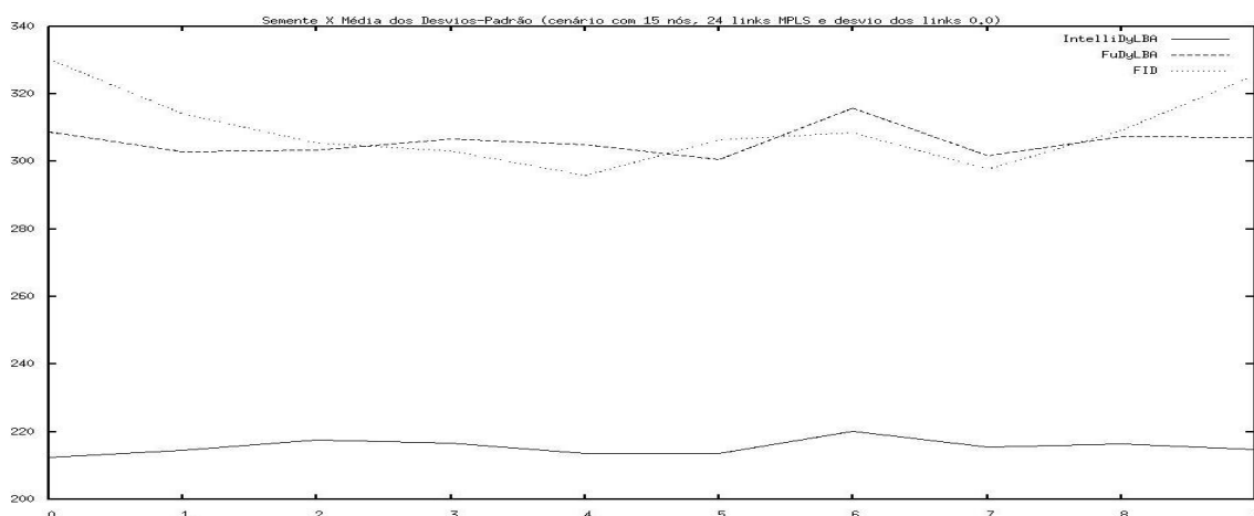
Figura 5.3. Média dos desvios padrão das bandas residuais dos enlaces ao longo dos experimentos da topologia 1.
